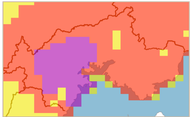
3時間後予測
